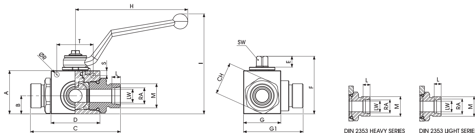
DIN 2353 HEAVY SERIES
